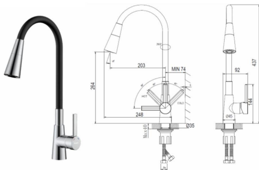
Смеситель для кухни с гибким изливом, Цвет черный/хром Z35-39-Black
