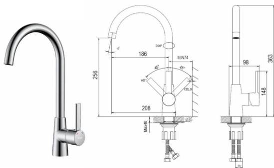
Смеситель для кухни с поворотным изливом Z35-40
