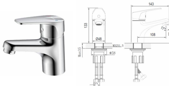
Смеситель для умывальника монолитный D40-13
