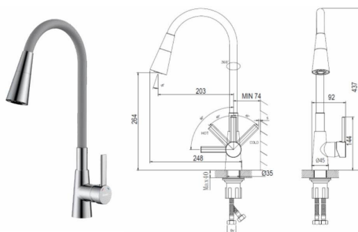
Смеситель для кухни с гибким изливом Цвет серый/хром Z35-39-Gray
