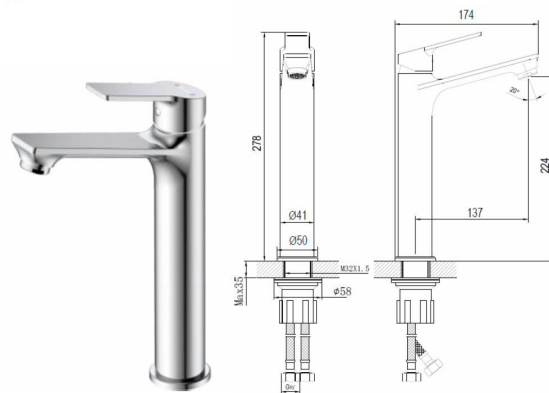
Смеситель для умывальника монолитный RS29-14
