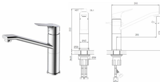
Смеситель для кухни с поворотным изливом RS29-25
