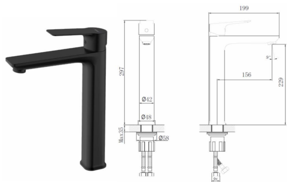
Смеситель для умывальника монолитный, черный RS27-14BL
