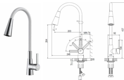
Смеситель для кухни с гибким изливом Цвет белый/хром Z35-39-White
