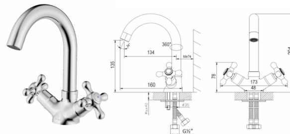
Смеситель для умывальника с поворотным изливом H02-64
