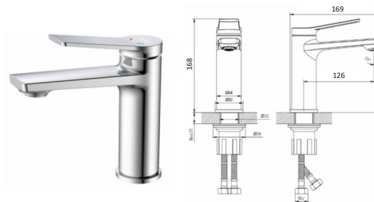
Смеситель для умывальника монолитный D40-13
