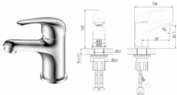
Смеситель для умывальника монолитный A35-13
