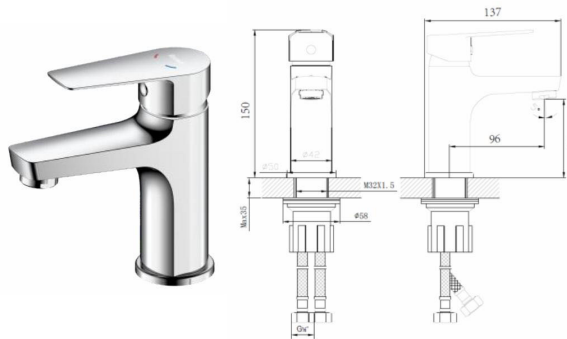
Смеситель для умывальника монолитный S35-13
