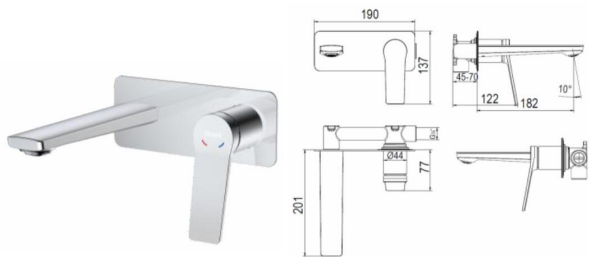
Смеситель для умывальника встраиваемый RS20-16
