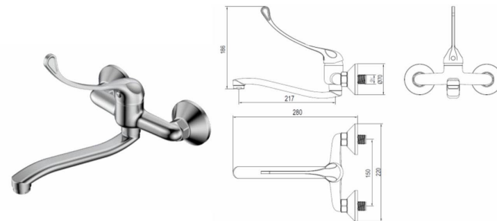
Смеситель для кухни и умывальника, настенный с нижним изливом, с локтевой рукояткой Y35-24
