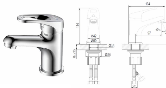
Смеситель для умывальника монолитный B35-13
